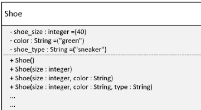
Abb: UML-Klassendiagramm mit überladenen Konstruktoren
