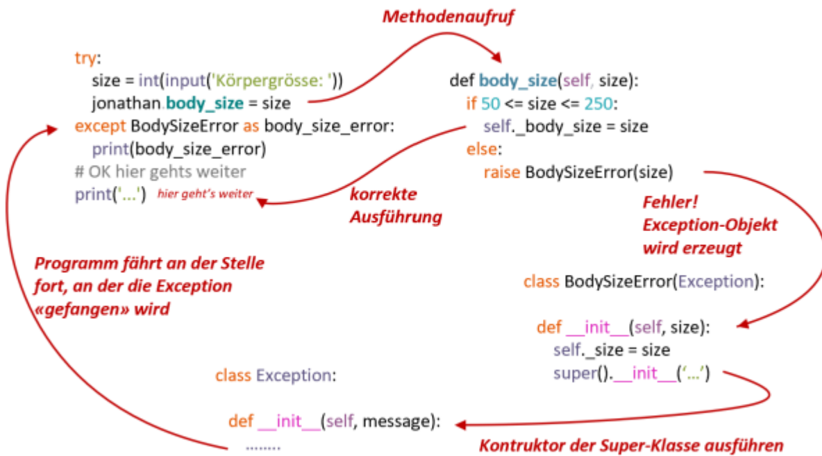
Abb: Ablauf bei einer Exception
