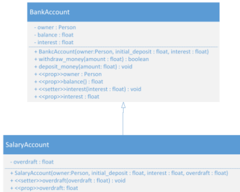
Abb: Unterklasse SalaryAccount
