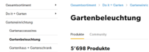
Abb. 1-10: hierarchische Darstellung
