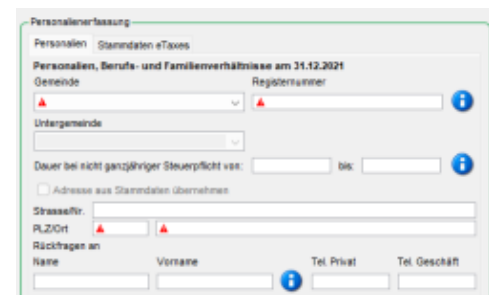
Abb. 1-11: tabellarische Darstellung
