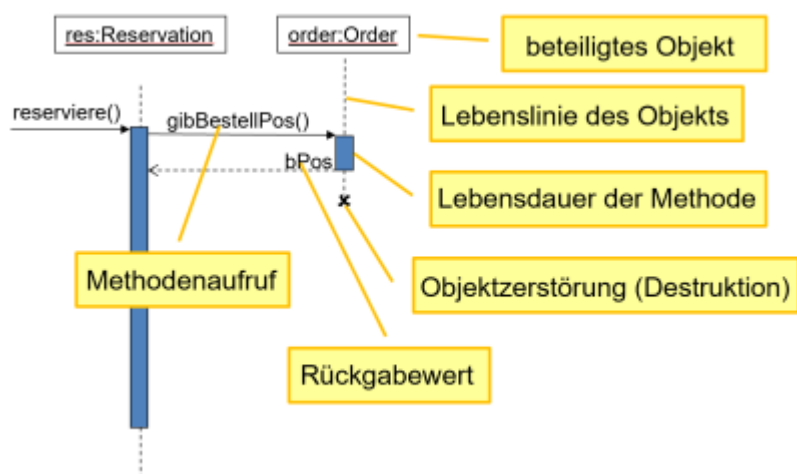
Abb 4.4: typische Elemente des Sequenzdiagramms
