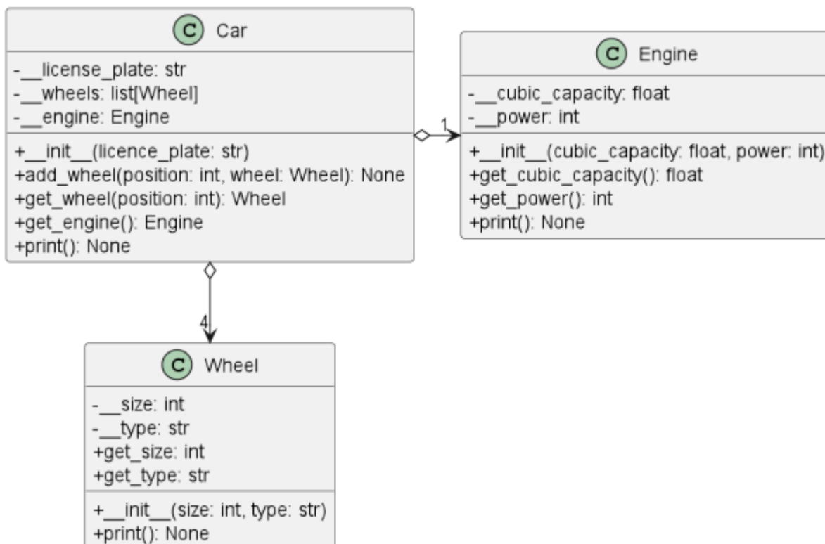
Abb. 1: Klassendiagramm
