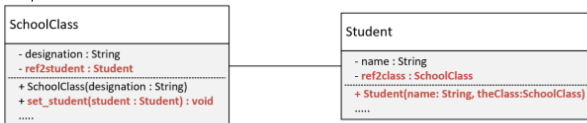
Abb 5.7: Klassen in einer zweiseitigen Beziehung
