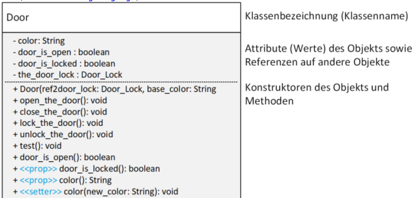
Abb: Klassendiagramm nach UML
