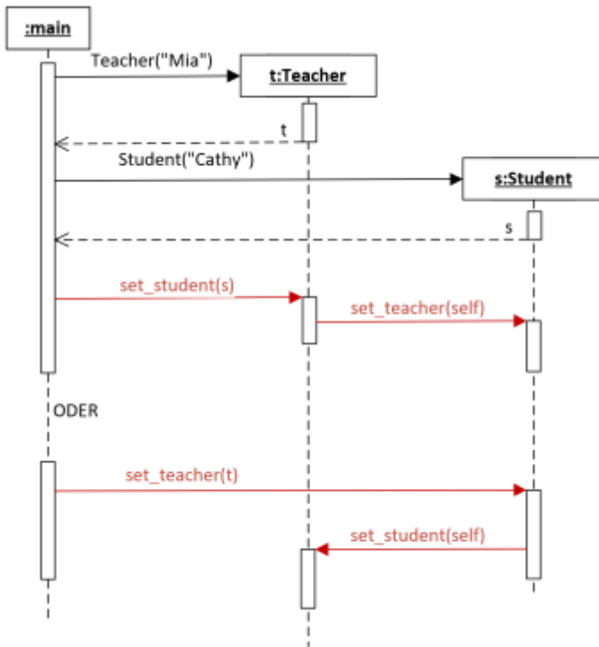
Abb: Sequenz-Diagramm der Zuweisung einer zweiseitigen Beziehung über Methoden
