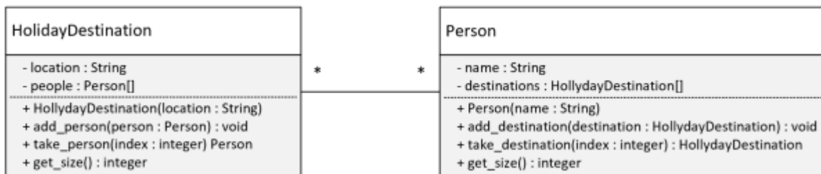
Abb 5.10 : n:n Beziehung
