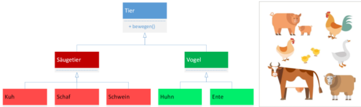
Abb 6.10: Vererbungshierarchie „Tiere“
