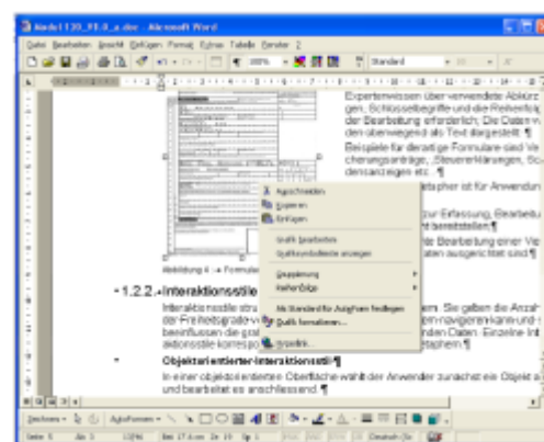
Abb. 1-5: Objektorientiertes GUI
