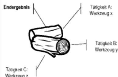
Abb. 1-4: Werkzeug-Material-Metapher
