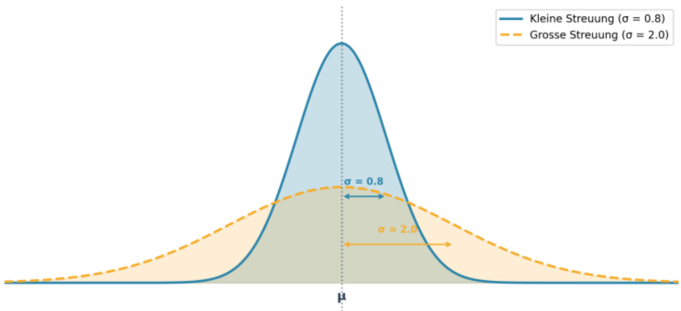
Standardabweichung - Kleines vs. grosses \sigma
